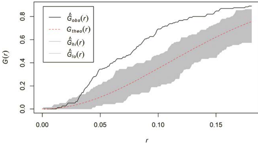
Abb. 6: Monte-Carlo-Simulation für Distanzen zur nächsten Nachbarburg
