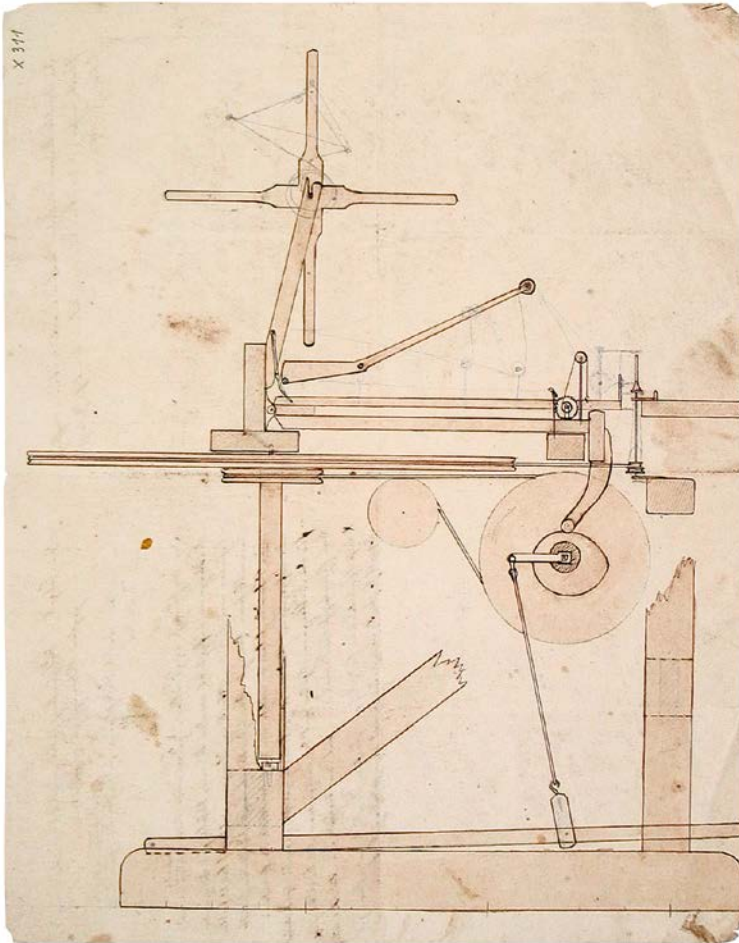
Abb. 3: Die Spulmaschine für Baumwollschussgarn für einen Baumwollzeugfabrikanten wurde mutmaßlich auf der Osnabrücker Gewerbeausstellung von 1838 gezeigt. Entwurf, Instrumentenmacher Kehlmann, Badbergen, 26. Februar 1838 (40 x 31,5 cm) (© Museumsquartier Osnabrück – Kulturgeschichtliches Museum, X 311)
